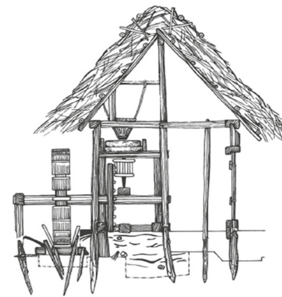
A: Reconstructie van een Karolingische watermolen, uit de achtste of de negende eeuw. 37 Tekening: Wolfgang Czynsz, Bayerisches Landesamt für Denkmalpflege.
